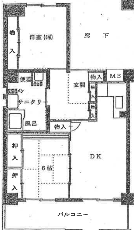
市営北柏B棟 (2DK-B)
