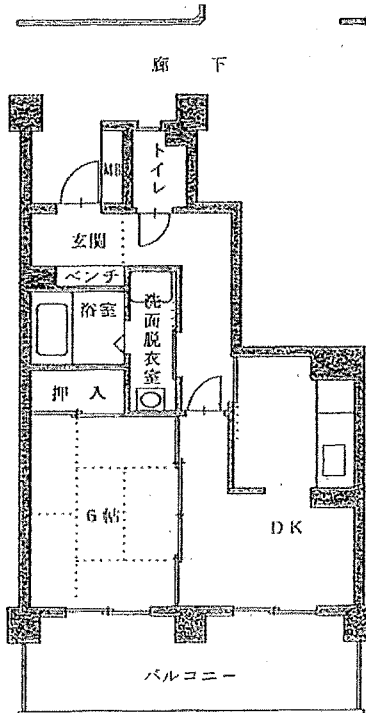
市営北柏E棟 (1DK) シルバー専用住戸
