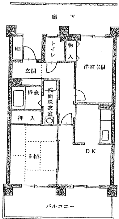
市営北柏E棟 (2DK) 一般住戸
