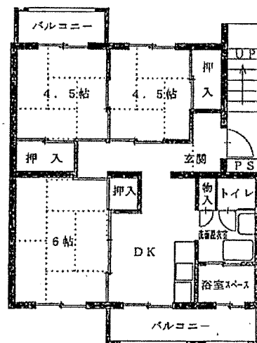
9 高田団地 (3DK) 10~12号棟 (反転あり)
