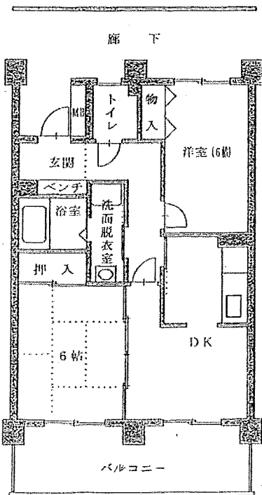
市営北柏E棟 (2DK) シルバー専用住戸
