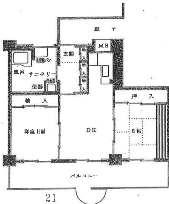
市営北柏B棟 (2DK-A)
