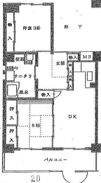
市営北柏B棟 (2DK-B)
