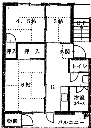
根戸団地 (3K) 8号棟 (反転あり)
