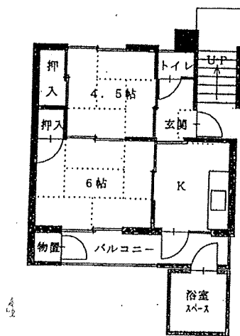
改良住宅団地 (2K) 1~4号棟 (反転あり)
