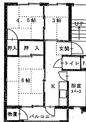
根戸団地 (3K) 6~7号棟 (反転あり)
