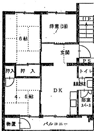
宿連寺団地 (3DK) 9号棟 (反転あり)
