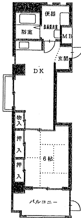
市営北柏B棟 (1DK-B) 単身者住戸 (反転あり)
