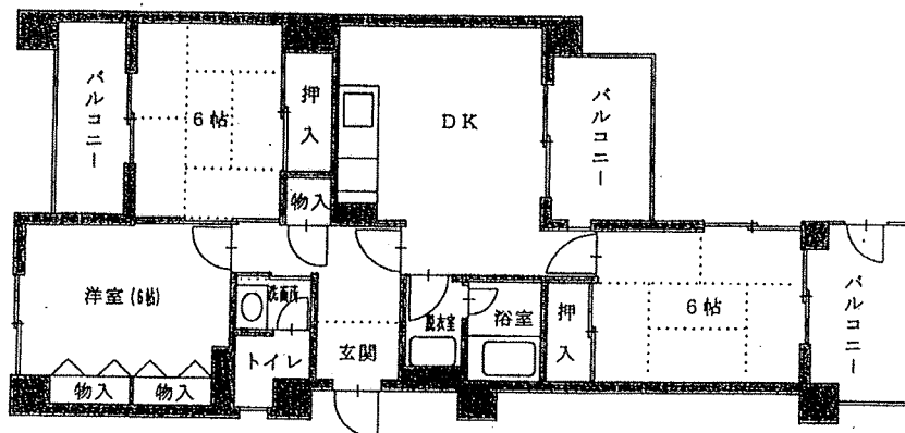
15 市営北柏A棟 (3DK-C)
